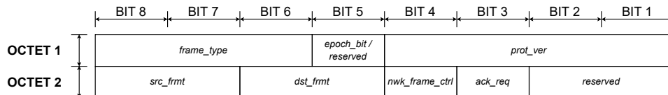
Fig. 5.36 Link layer - Message - Frame control
