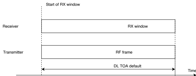
Fig. 5.43 No timedrift
