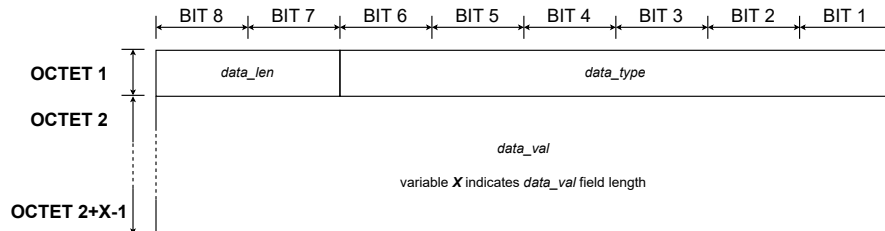
Fig. 5.32 Link layer - Beacon - Data - Case 1
